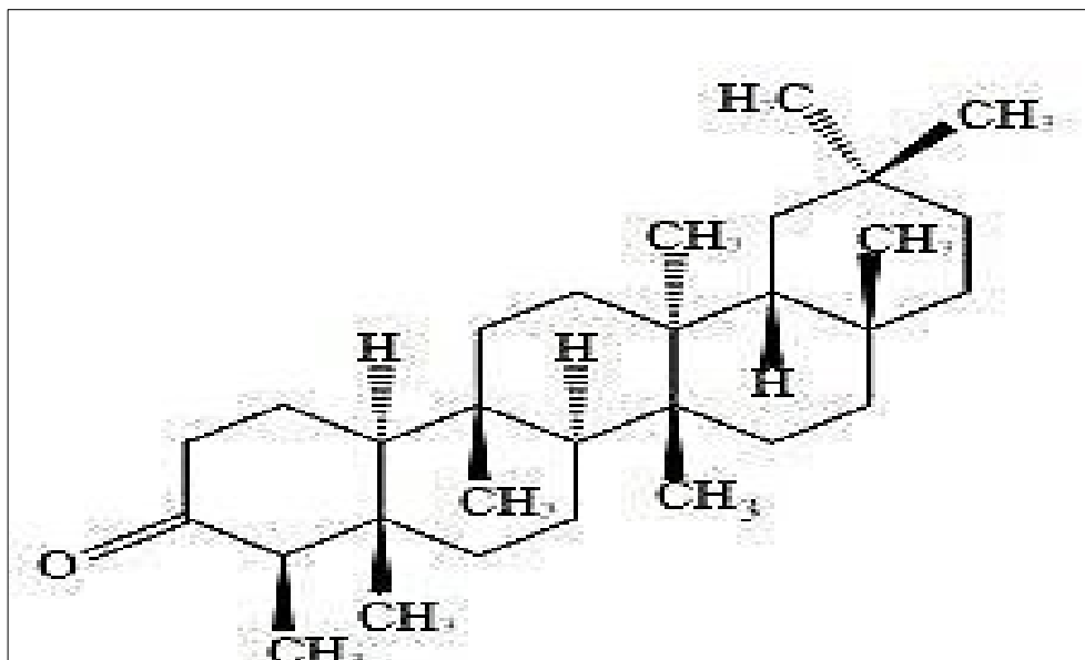
Fig 2: Friedelin
