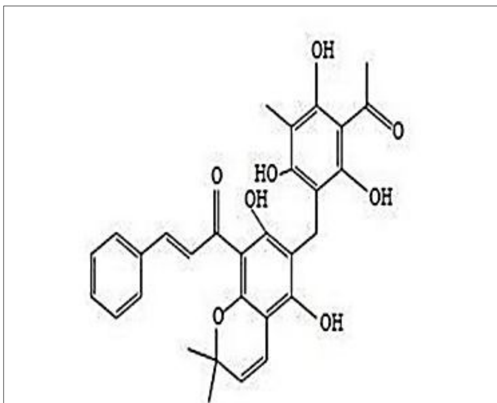
Fig 15; Rottlerin
