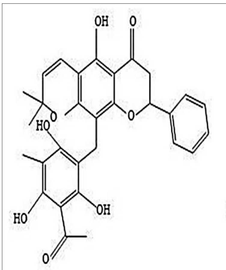
Fig 17: Isorottlerin
