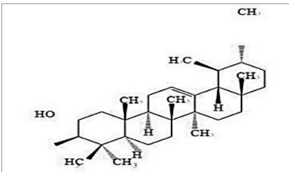
Fig 5: Amvrin
